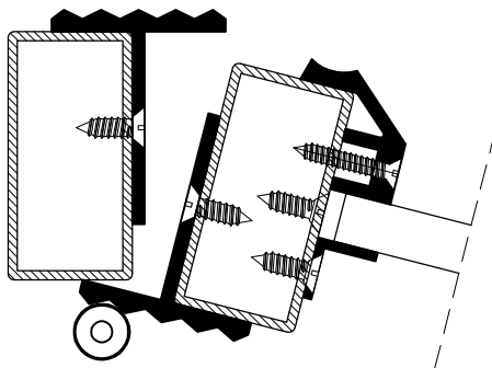
Otvoren položaj Open position
