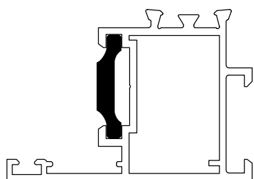
Pogonska letva za EURO1 žljeb EURO1-grooved sliding rod
