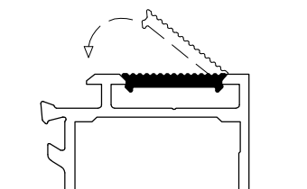
Čep praga za EURO1 žljeb EURO1-grooved threshold plug
