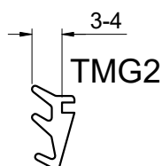
Zaptivke stakla Glazing gasket Прокладка стекла
