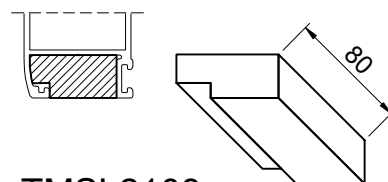
TMSL2108 Sunder - guma Sponge - gasket Губка - прокладка Za/for/Для: TMSL307
