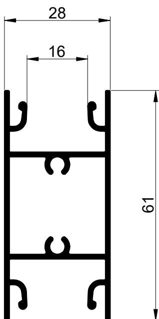
TMSL2009 0,845 kg/m`
