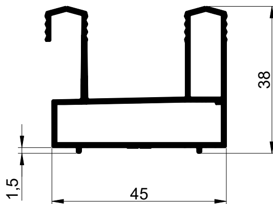
TMSL2001 0,742 kg/m`
