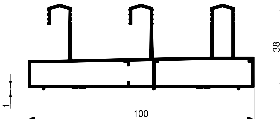
TMSL2002 1,340 kg/m`
