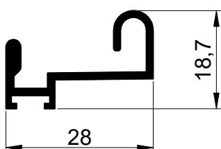
TMSL2012 0,270 kg/m`
