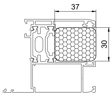
952 Penasti profil u krilu Foam profile in sash Пенный профиль в створке
