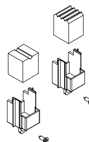
Čepovi za središnja krila Plugs for central sash Заглушки для центральной створки
